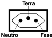
Figura 4: Tomada modelo nacional com fio terra
