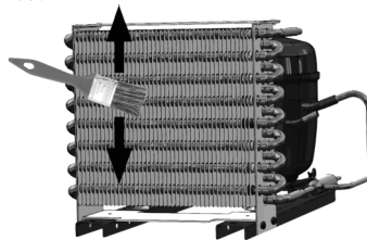
Figura 12: Limpando o condensador
